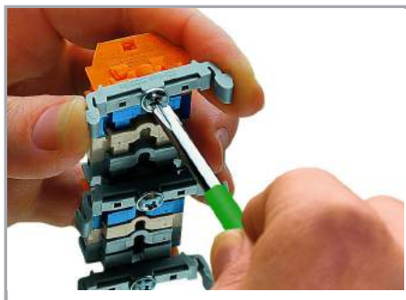
Listwa zaciskowa; z uchwytami montażowymi,
