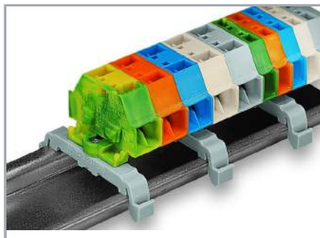
Listwa zaciskowa; z uchwytami montażowymi; na szynie TS 35
