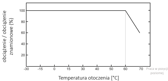
CHARAKTERYSTKA OBCIĄŻALNOŚCI W ZALEŻNOŚCI OD TEMPERATURY OTOCZENIA
