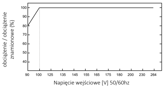
CHARAKTERYSTKA OBCIĄŻALNOŚCI W ZALEŻNOŚCI OD NAPIĘCIA WEJŚCIOWEGO
