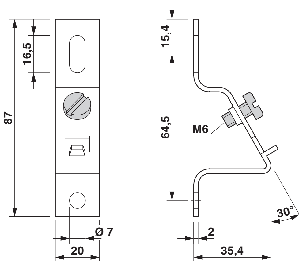
Rysunek wymiarowy
