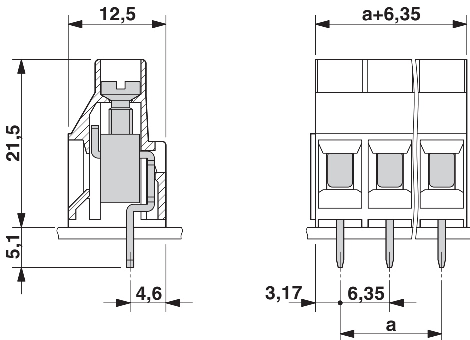
Rysunek wymiarowy
