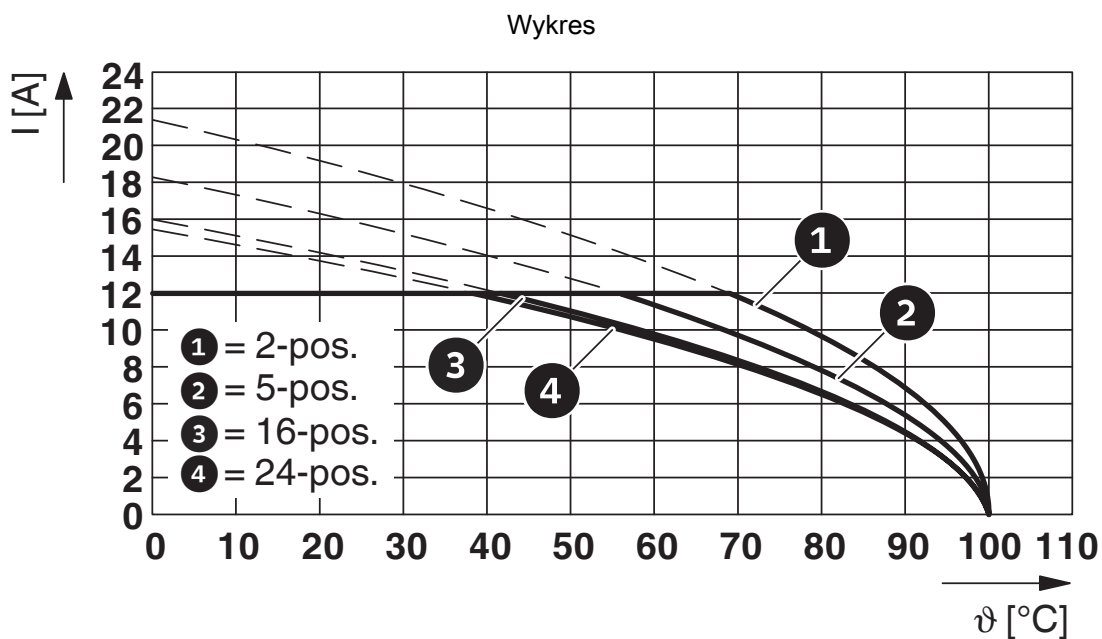
Typ: SMSTB 2,5/...-STF z MSTB 2,5/...-GF-5,08
