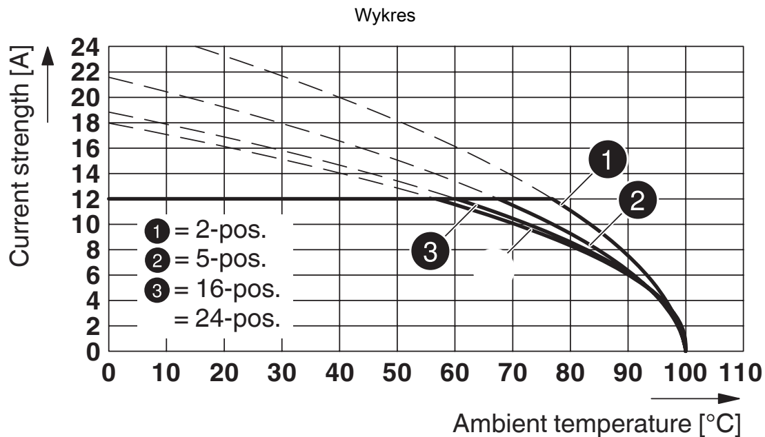
Typ: FRONT-MSTB 2,5/...-STF-5,08 z MSTB 2,5/...-GF-5,08
