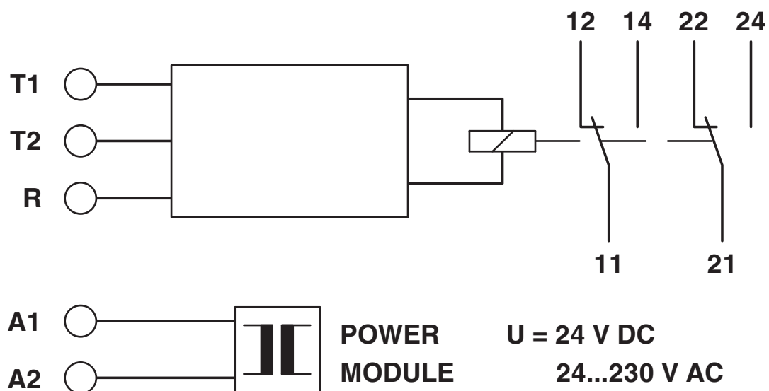
Schemat blokowy
