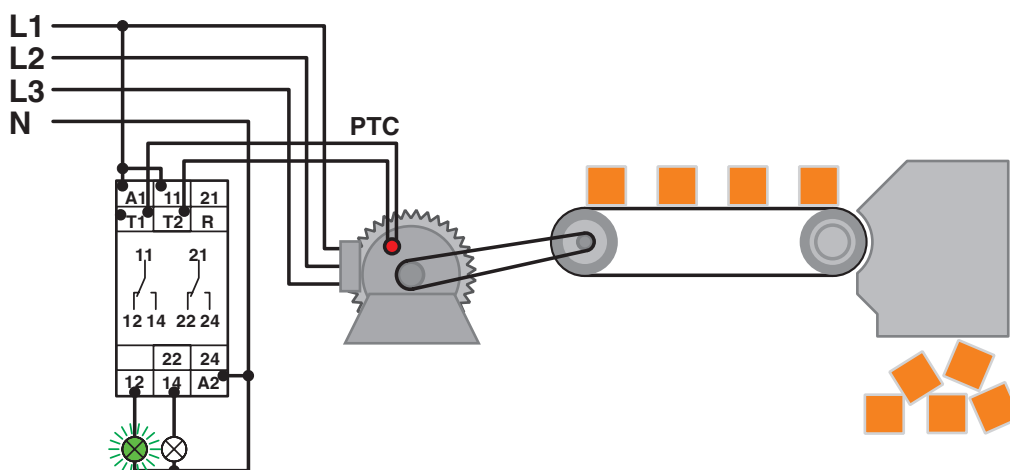
rysunek aplikacji
