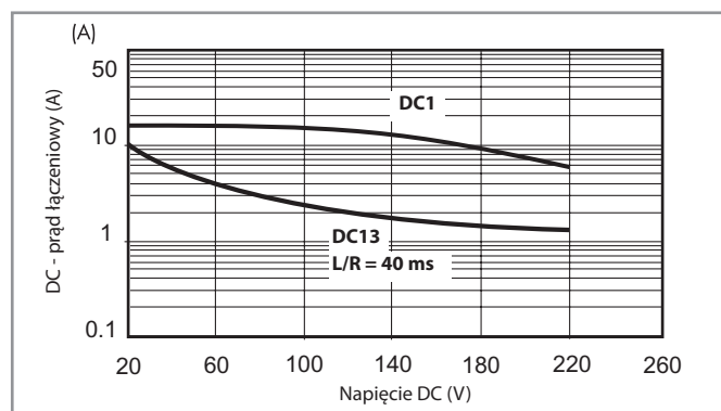
H 62 - Obciążenie graniczne dla prądu stałego 62.32.9.xxx.4800
