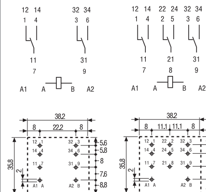
62.22 Rysunek otworów montażowych
