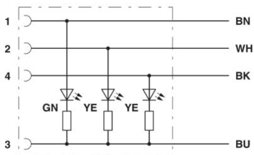
Kontaktbelegung des M12-Steckers und der M12-Buchse, mit LED
