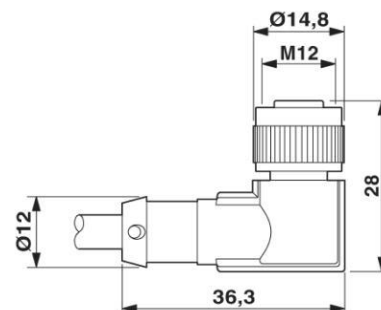
Buchse M12 x 1, gewinkelt, mit LED
