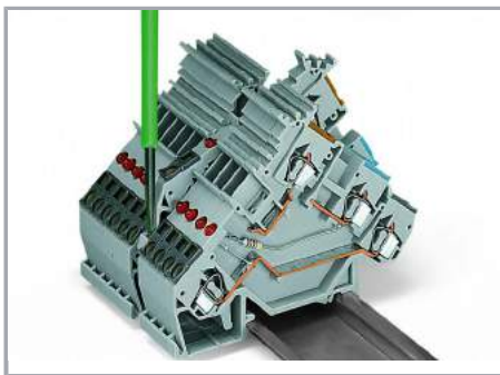
Demontaż z szyny montażowej. Uwaga – należy uprzednio usunąć mostki!
