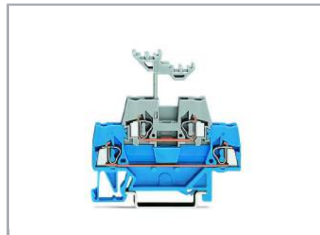
Złączki dwupiętrowe łączą w jednej obudowie izolacyjnej dwie złączki o różnych potencjałach, ustawione piętrowo – jedna nad drugą, przy czym kolory poszczególnych pięter mogą być takie same lub – jak w przypadku serii 280 – różne. Dolne piętro złączki jest szersze, co znacznie ułatwia montaż i demontaż przewodów.
