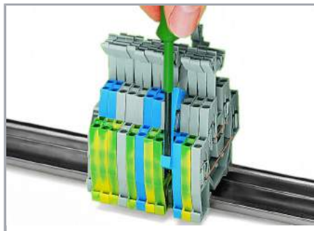
Demontaż pojedynczej złączki z listwy zaciskowej
