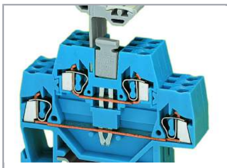
Mostkowanie przy użyciu mostka pionowego (281-421)
