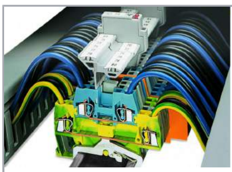
Przykład listwy zaciskowej złożonej ze złączek dwupiętrowych różnego typu
