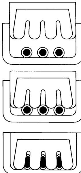
Prinzipdarstellung einer Kontaktierung
