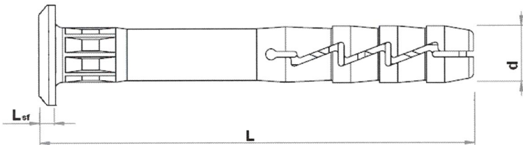
Tuleja FX-..K..
