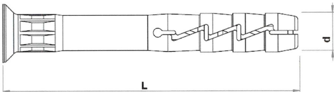
Tuleja FX-..L..
