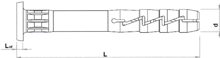
Tuleja FX-..C..
