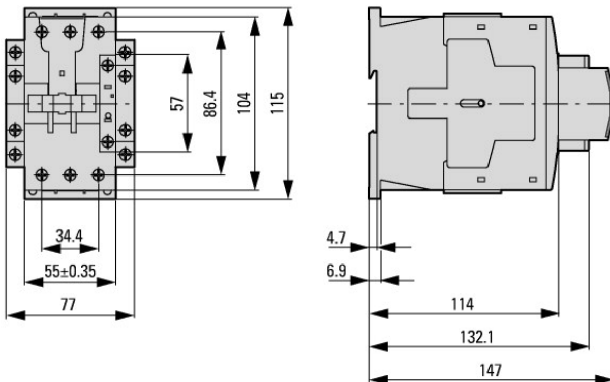
Stycznik z modułem styków pomocniczych
