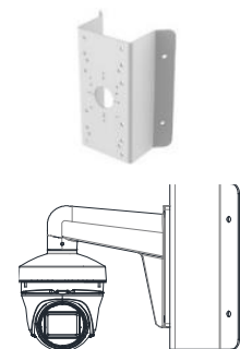
DS-1276ZJ-SUS Mocowanie narożne
