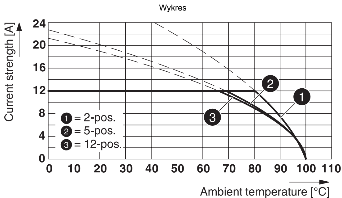
Typ: FKCN 2,5/...-ST-5,08 z MSTBA 2,5/...-G-5,08
