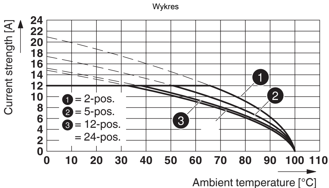
Typ: MVSTBR 2,5/...-ST-5,08 z MSTBA 2,5/...-G-5,08
