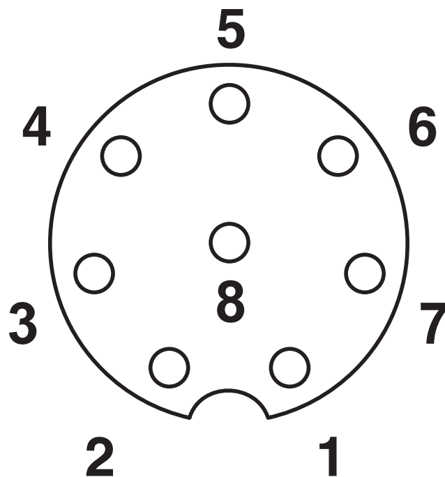
Rysunek schematyczny
