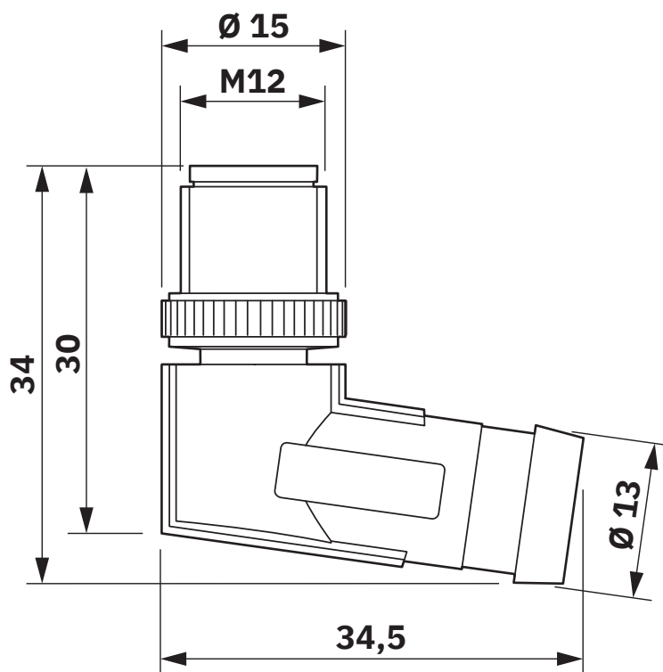
Rysunek wymiarowy
