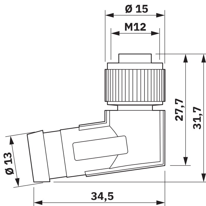
Rysunek wymiarowy
