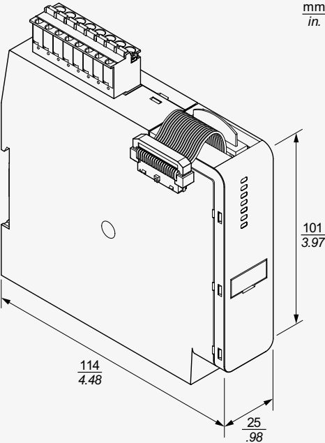
Digital I/O module: TPRDG4X2
